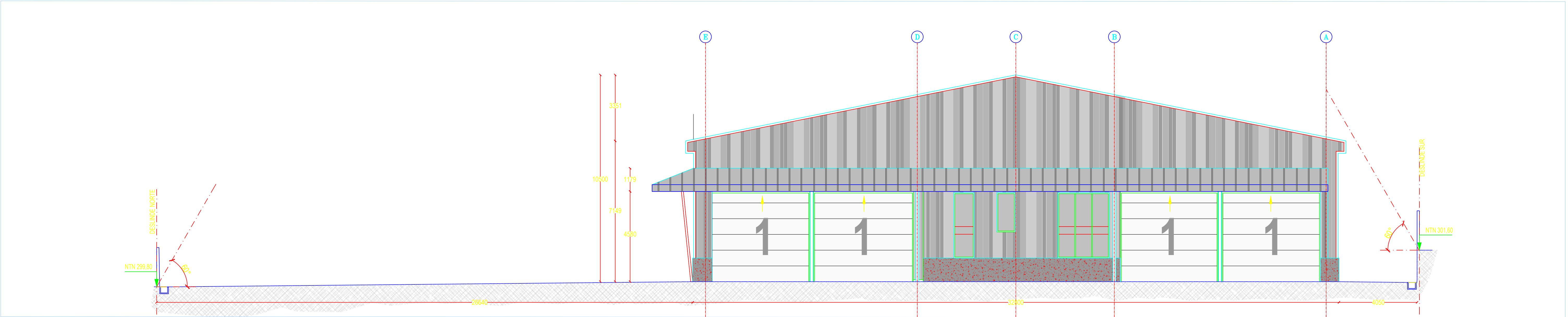
ELEVACIÓN PONIENTE PROPUESTA MODIFICACIÓN PON N° 47 DEL 08/04/2026 ESCALA 1:100
